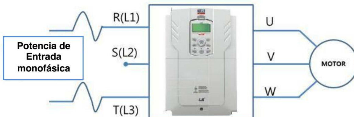
Figura-3 Diagrama de Conexionado de Bornes
